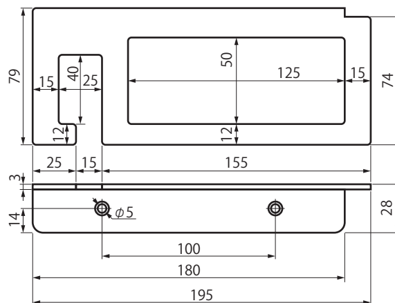
寸法図 (mm)
