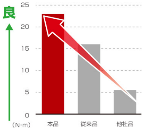
ドリルの滑り始めトルク比較
