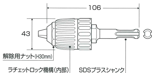
ラチェットロック機構(内部)
