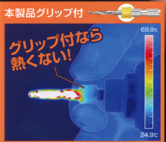
硬木への穴あけ後のサーモグラフィ比較
