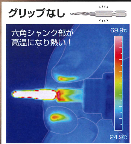
硬木への穴あけ後のサーモグラフィ比較
